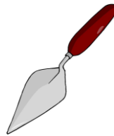
la truelle
