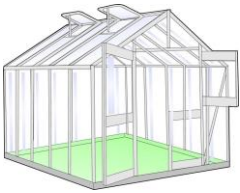
la serre
